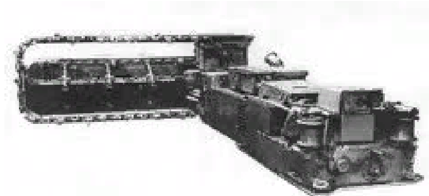
Очистной комбайн типа «Донбасс», сконструированный на основе изобретения А. Бахмутского
