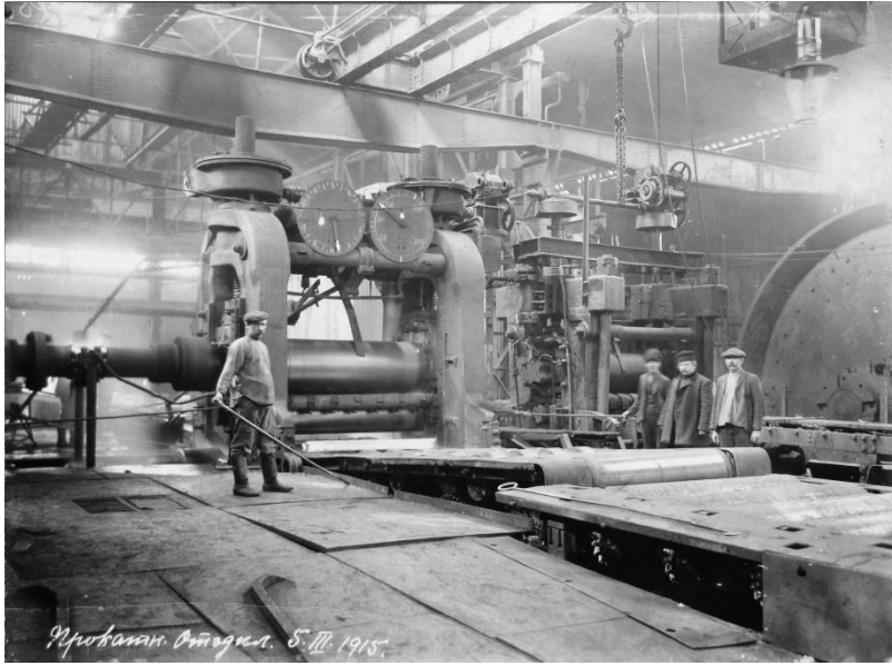
В листопрокатном цехе завода Новороссийского общества, 1915 г.
