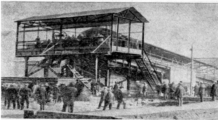
Первая отечественная разливочная машина, г.Енакиево, 1931 г.
